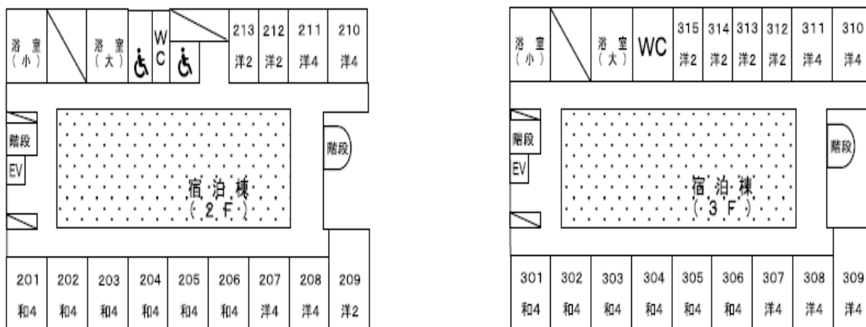
〔宿泊棟平面図〕
